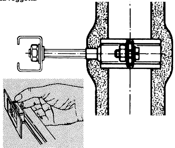
Targhetta universale senza reggetta
