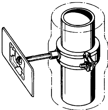
Targhetta da avvitare
